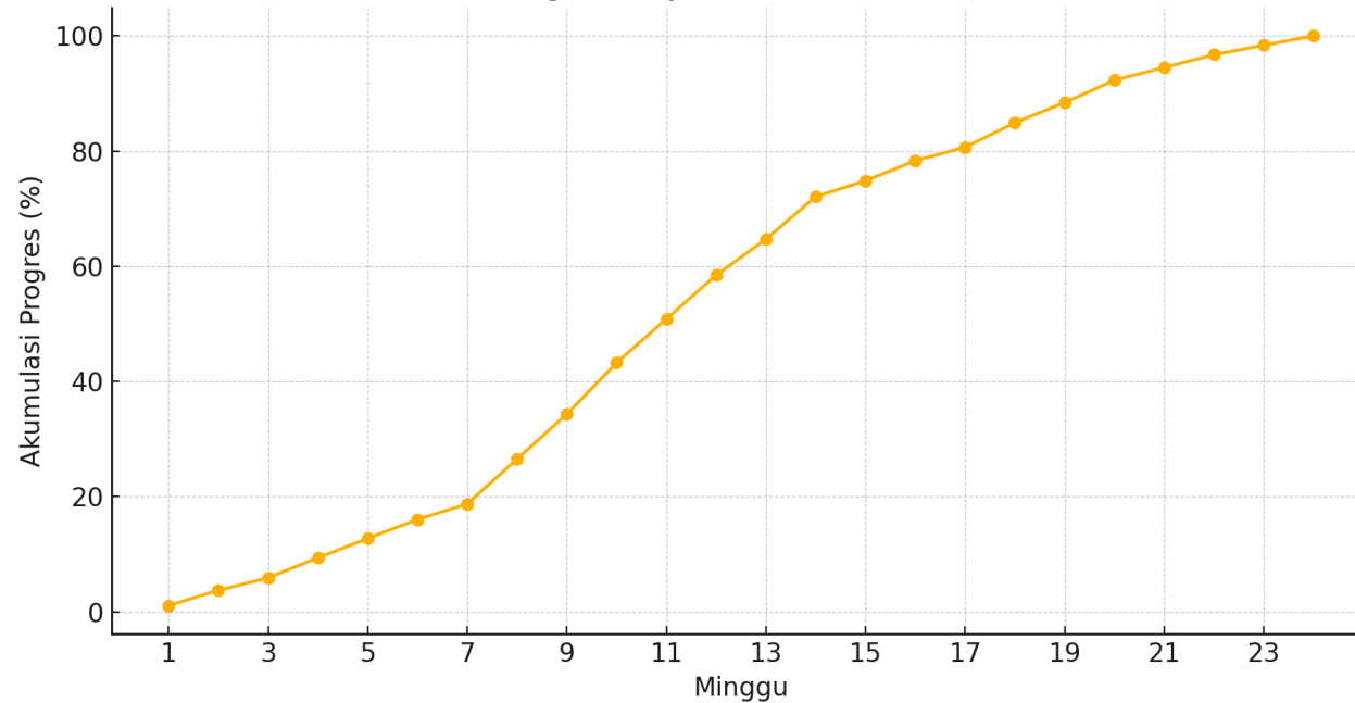
Kurva S Progres Proyek Rumah 2 Lantai Pak Amir
